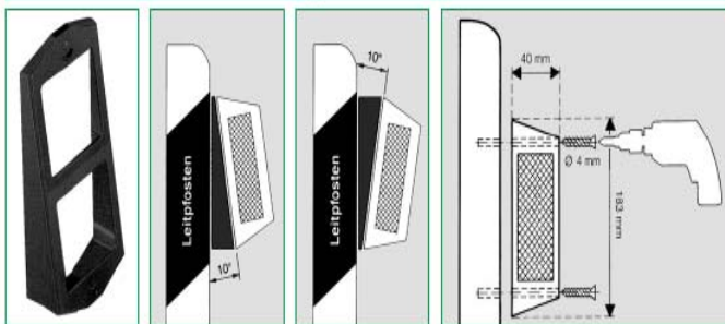
Montage Keil Bestell-Nr.: 790 302
